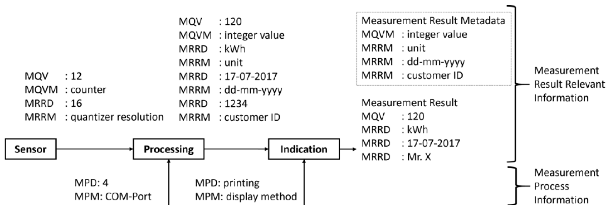
Obr. A.2 – Vývojový diagram procesu měření s příklady pro různá data související s výsledkem měření nebo relevantní pro proces měření.
